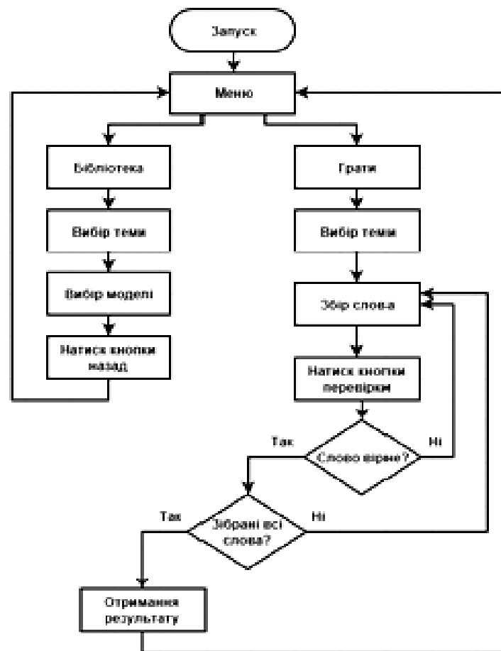
Рис. 10. Алгоритм програми
